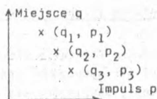
Rys. 1. Stany jako punkty w przestrzeni fazowej
