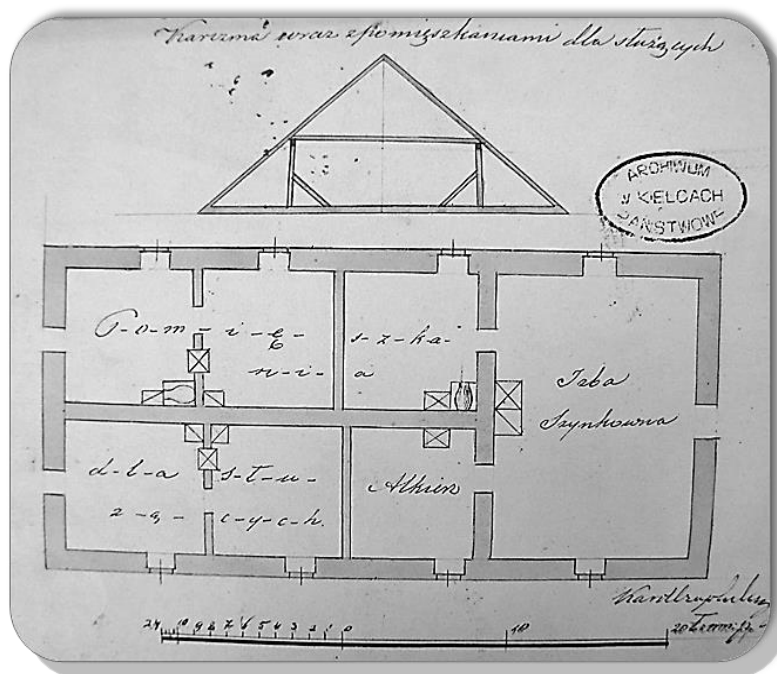
14. Rzut i przekrój poprzeczny dachu karczmy w Karsznicach, 1858 r.
