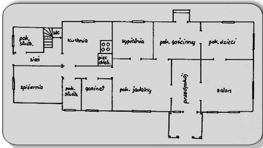
17. Rozkład pomieszczeń dworu w Mieronicach
