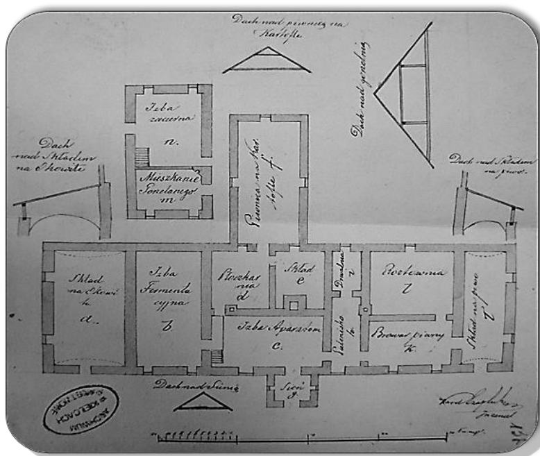
10. Rzut i przekrój dachu gorzelnii w Rembieszycach, 1862 r.
