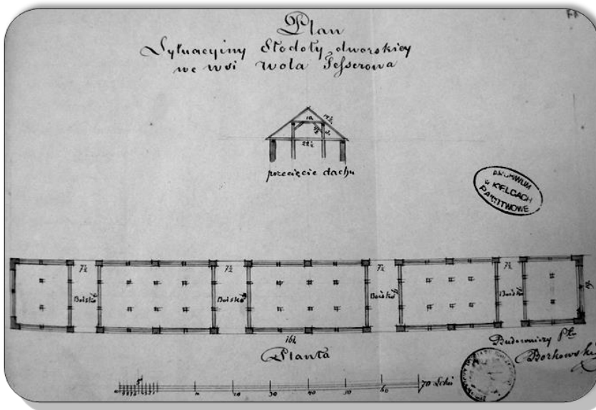
22. Plan i przekrój dachu stodoły dworskiej w Woli Tesserowej, 1865 r.
