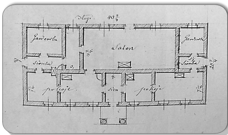
9. Plan sytuacyjny dworu w Rembieszycach, 1852 r.
