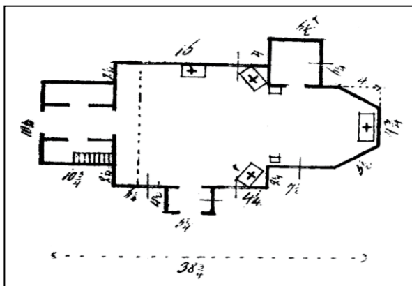
25. Plan kościoła w Rembieszycach, XIX w.
