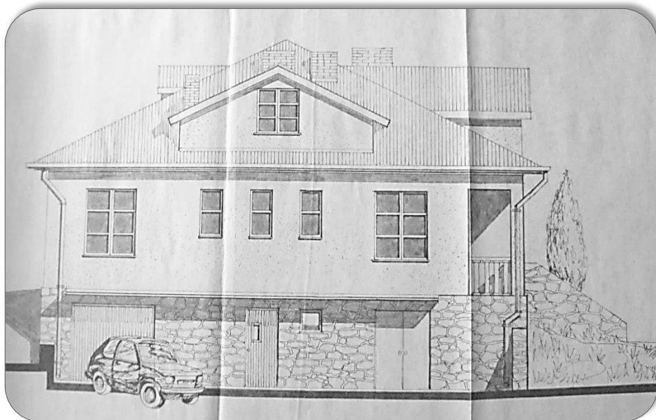
38. Elewacja wschodnia plebanii w Rembieszycach, projekt, 1984 r.
