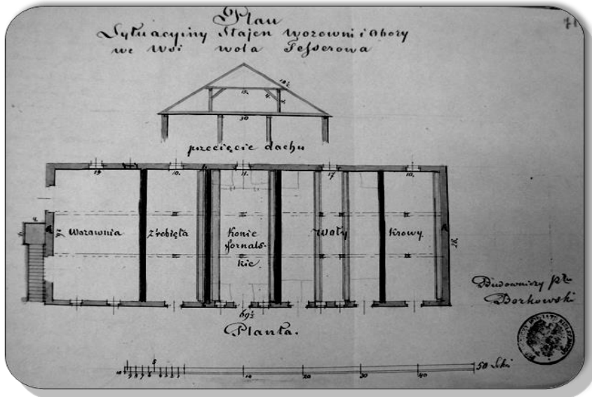
21. Plan i przekrój dworskich stajen, wozowni i obory w Woli Tesserowej, 1865 r.
