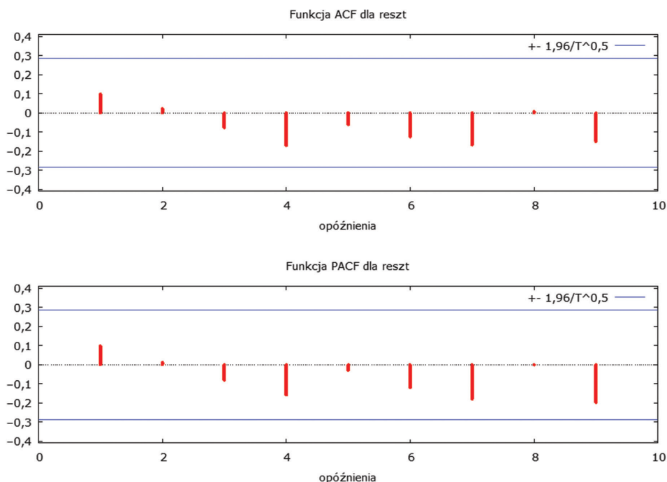
Wykres 43. Funkcja ACF i PACF dla reszt
