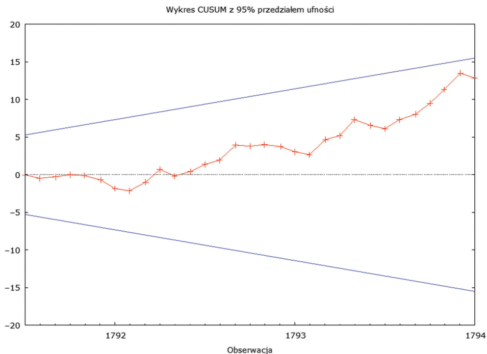
Wykres 38. Test CUSUM
