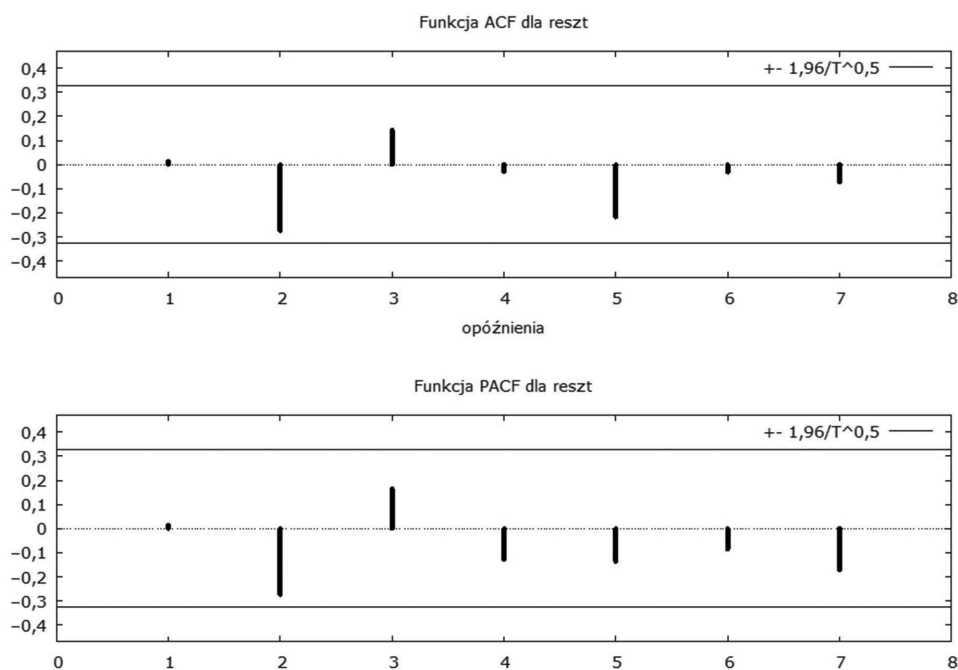
Wykres 36. Funkcja ACF i PACF dla reszt
