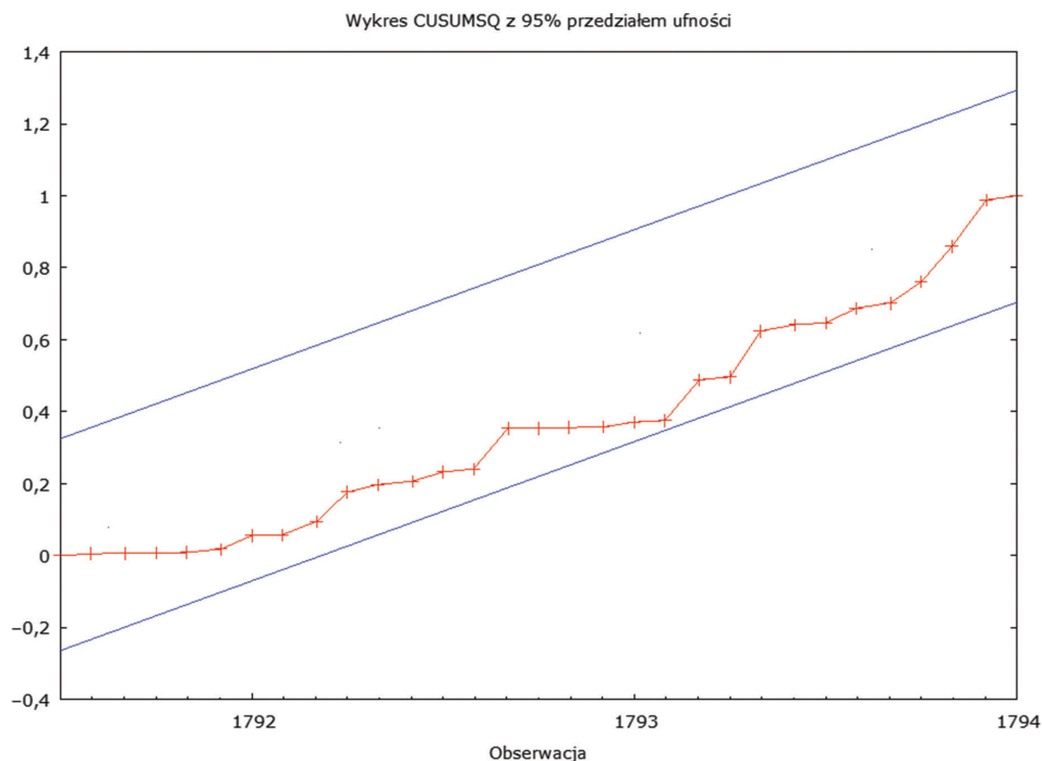
Wykres 39. Test CUSUMSQ
