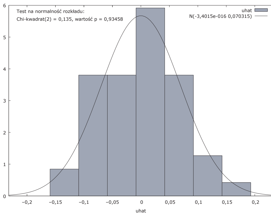
Wykres 44. Test Doornika-Hansena
