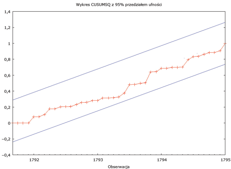
Wykres 46. Test CUSUMSQ
