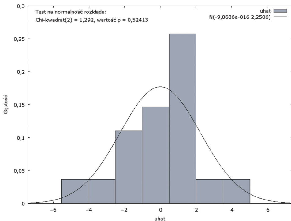
Wykres 37. Test Doornika-Hansena
